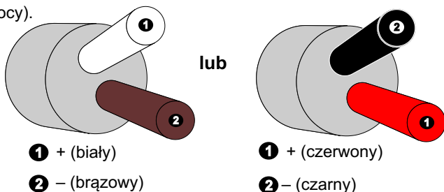
a) Schemat podłączenia lamp z driver'em napięciowym (np. PX254 lub PX282)
