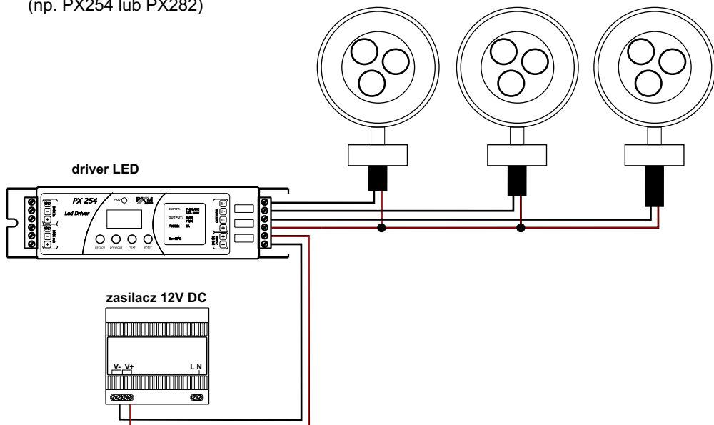
b) Schemat podłączenia lamp z zasilaczem
