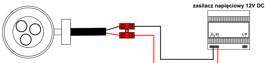
b) Schemat podłączenia lamp z zasilaczem
